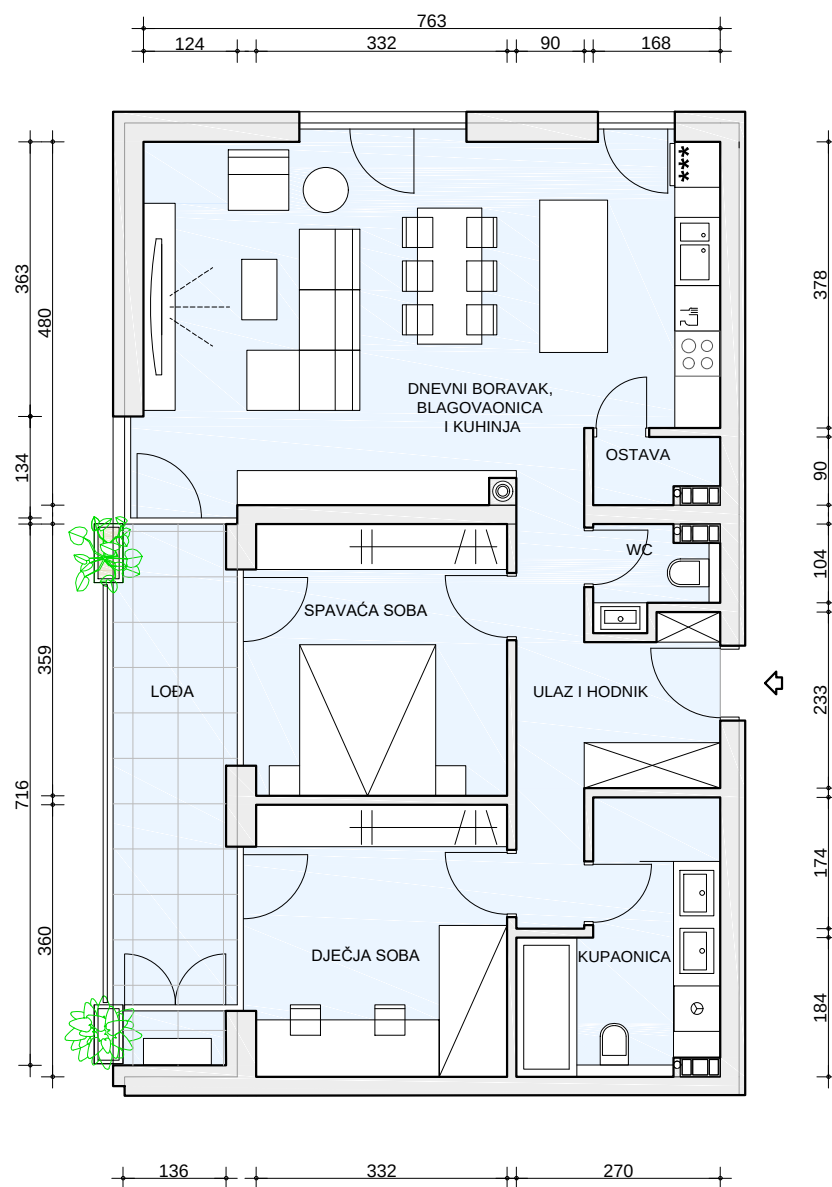
TLOCRT STANA MJERILO 1:100
