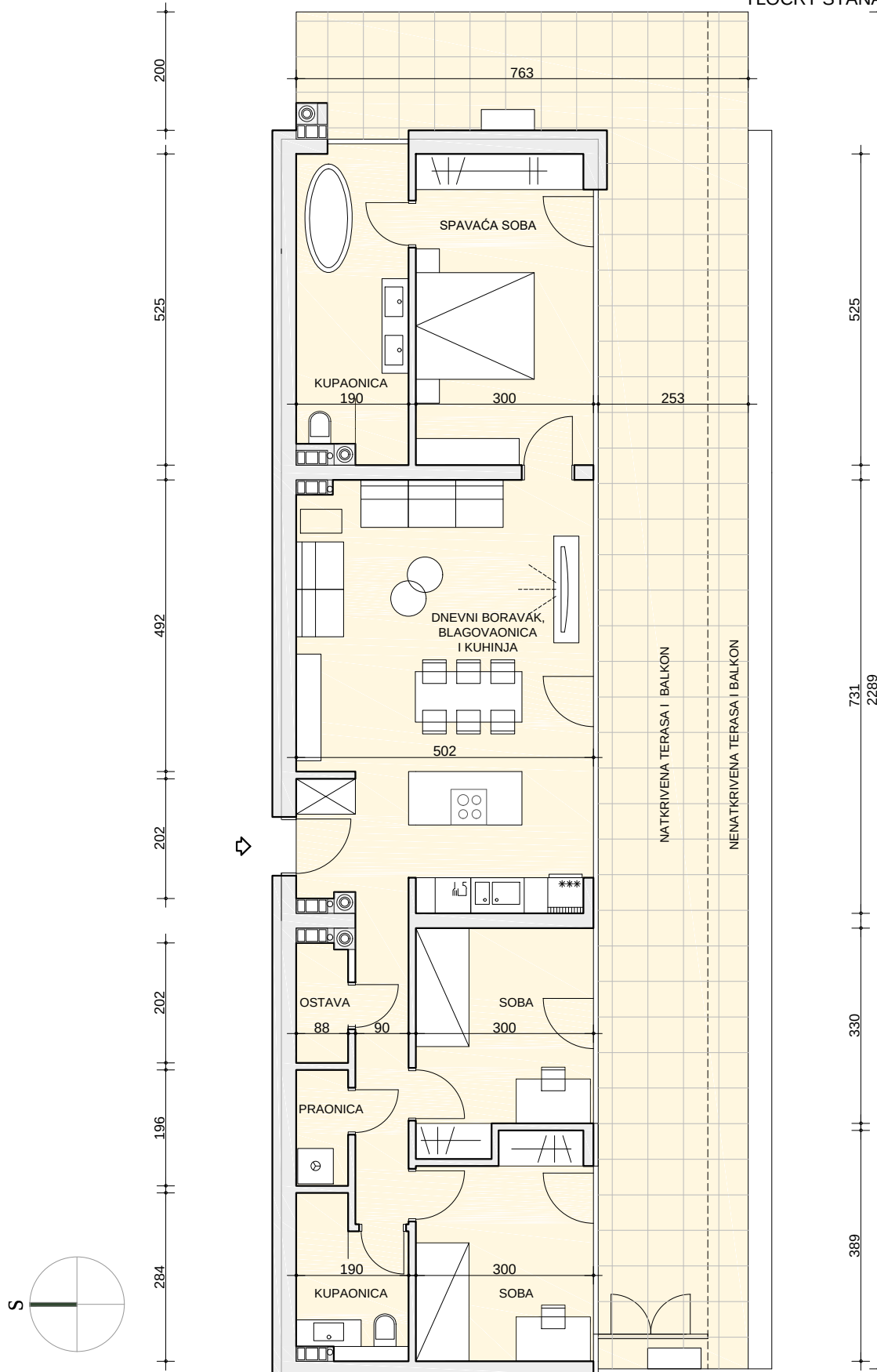
TLOCRT STANA MJERILO 1:100
