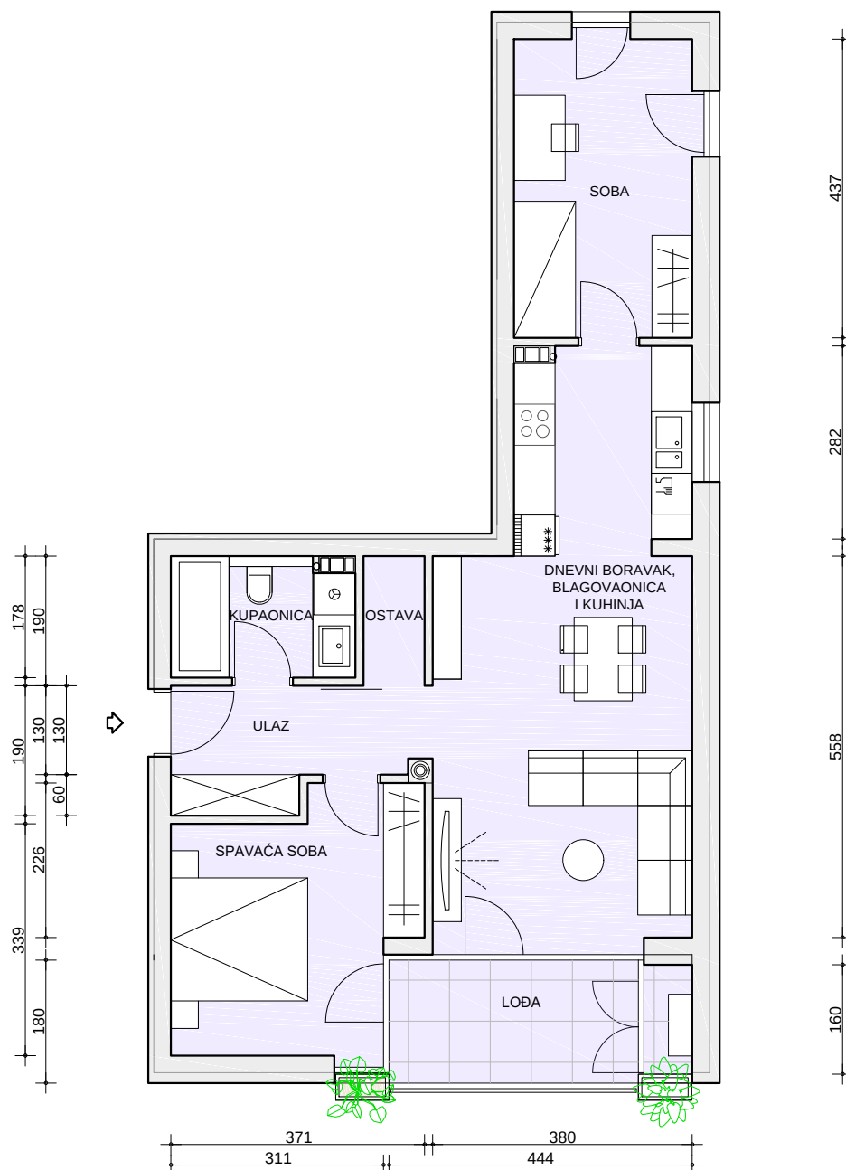
TLOCRT STANA MJERILO 1:100
