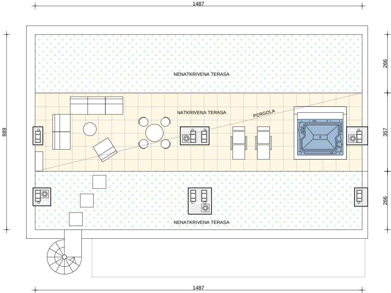
TLOCRT KROVA STANA MJERILO 1:100
