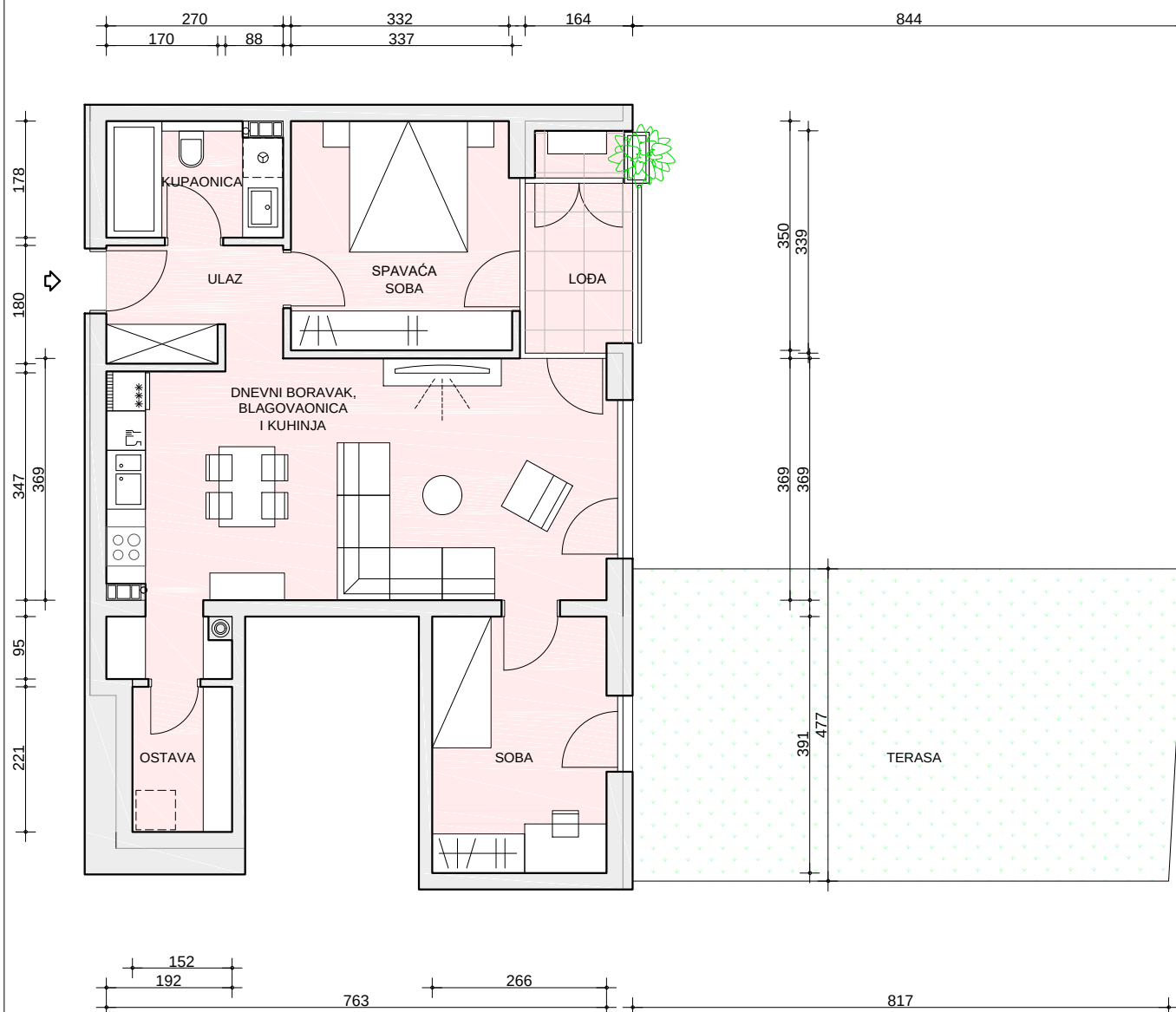
TLOCRT STANA MJERILO 1:100
