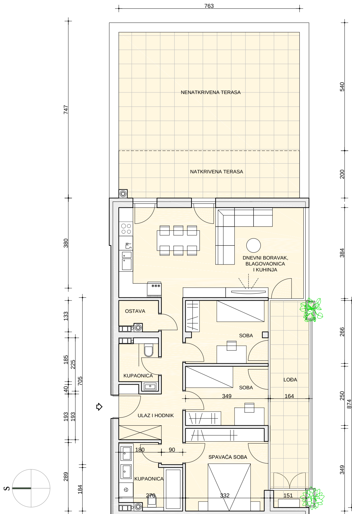
TLOCRT STANA MJERILO 1:100
