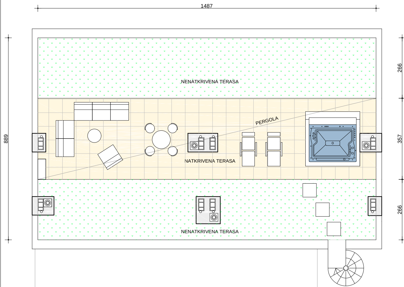
TLOCRT KROVA STANA MJERILO 1:100
