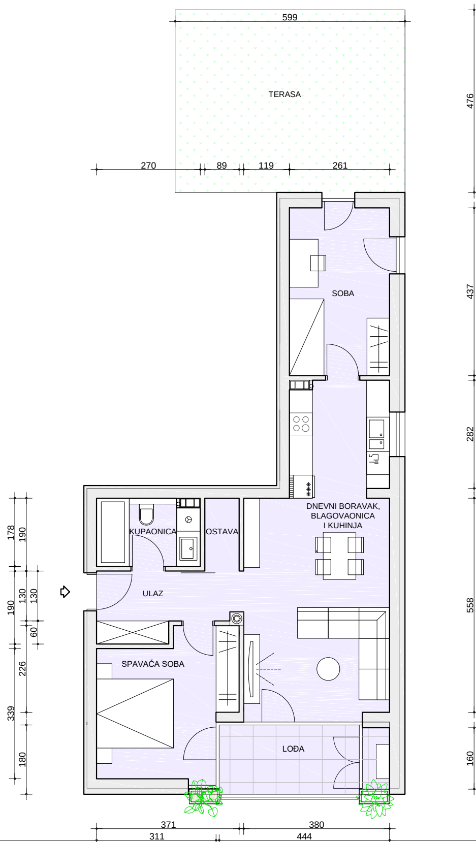
TLOCRT STANA MJERILO 1:100
