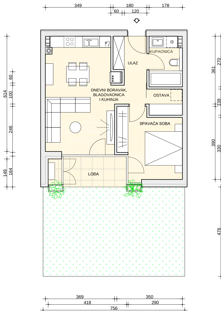
TLOCRT STANA MJERILO 1:100
